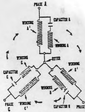
WANLASS MOTOR
