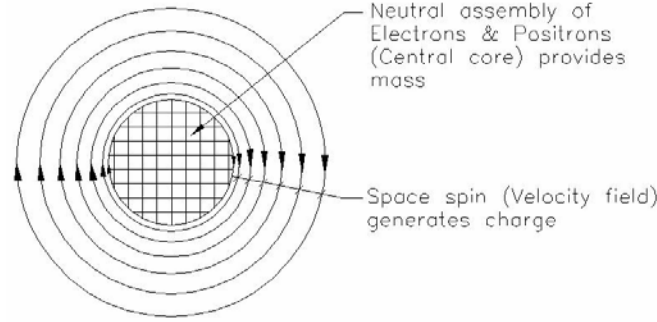
Fig. 10 Proton
