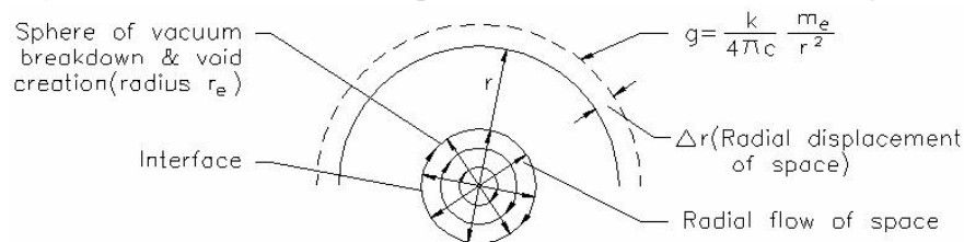
Fig. 6 Gravitation
