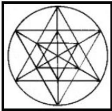
Fig. 11 - SP1 or Partiki Unit
